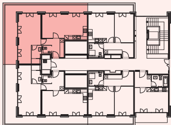
Schéma půdorys
